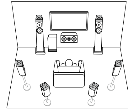
7.1.2 (Enceintes Dolby Activé (Avant ou Surround ou Surround arriere)) ( →p35)
