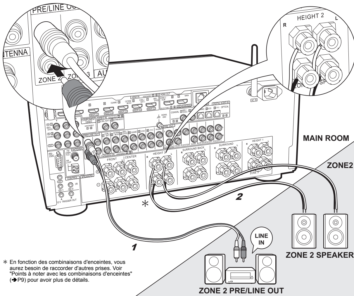
1 Câble audio analogique, 2 Câble d'enceinte
