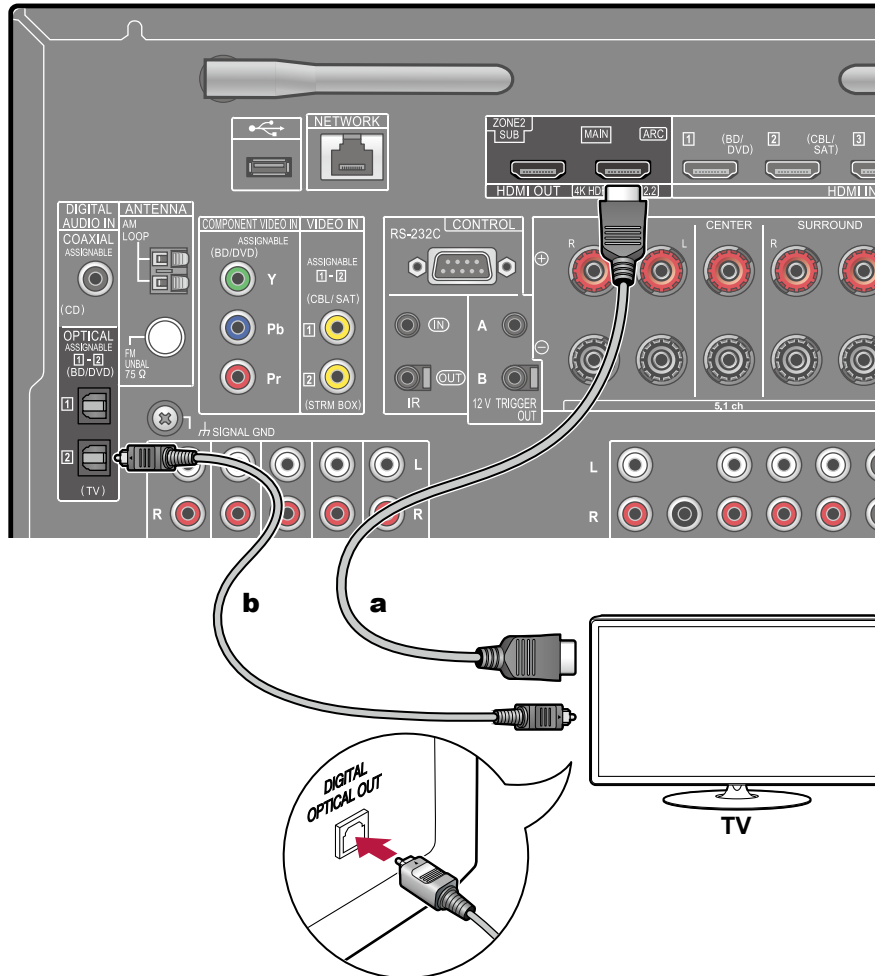
a Câble HDMI, b Câble optonumérique
