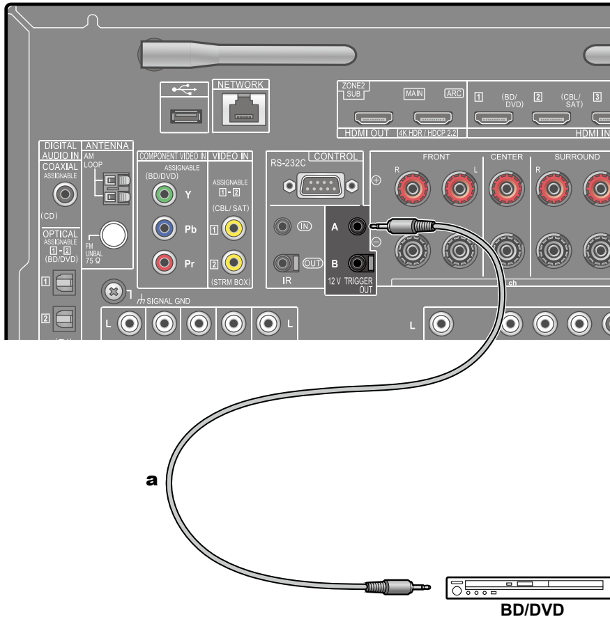
a Câble mini-prise monophonique (ø1/8"/3,5 mm)
